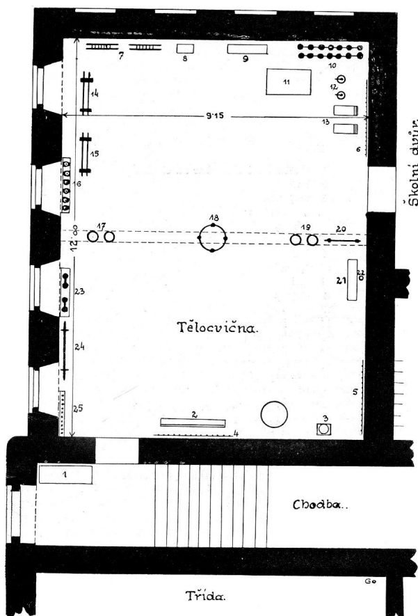
Plán školní tělocvičny.
