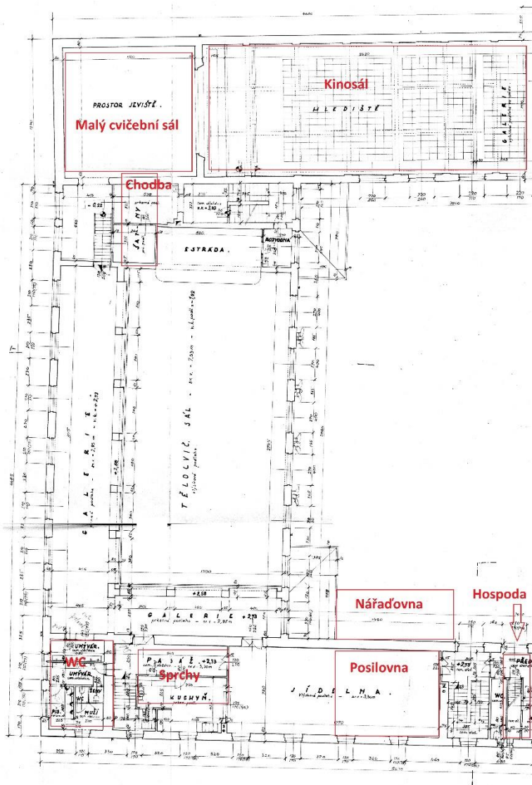
Obr. 10 Původní půdorys 1 NP sokolovny z 30. let 20. st. a současný stav
