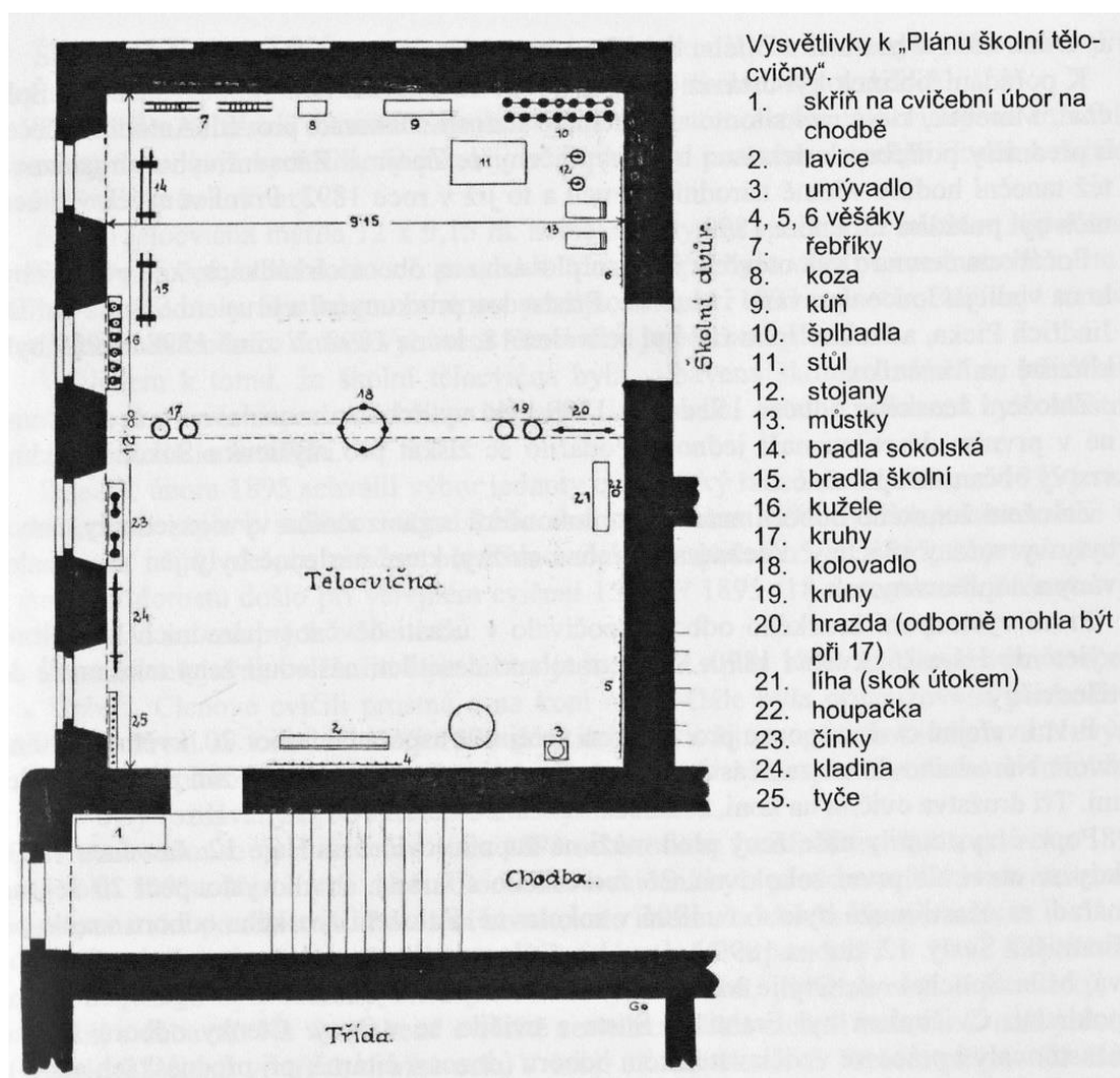
Obr. 3 Plán školní tělocvičny
